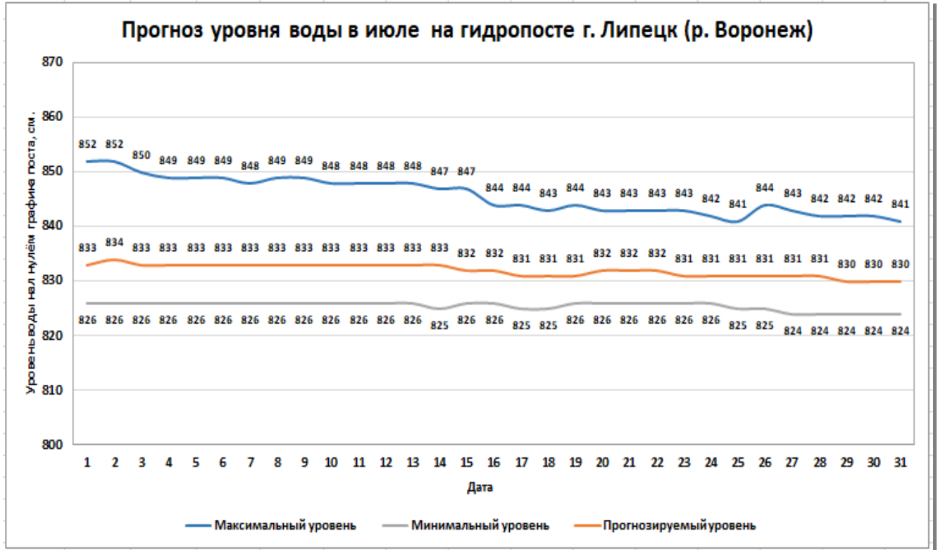
Рис. 9. Прогноз уровня воды в июле на гидропосте г. Липецк (р. Воронеж)
